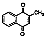
MENADIONE:
